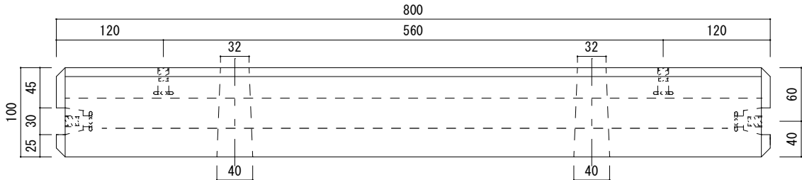
側面図
