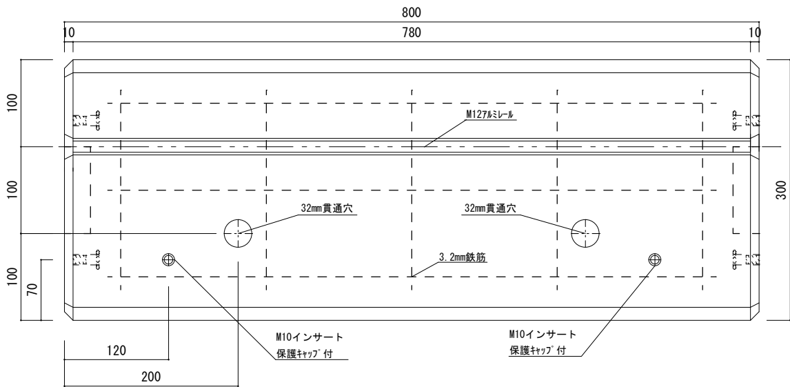
平面図
